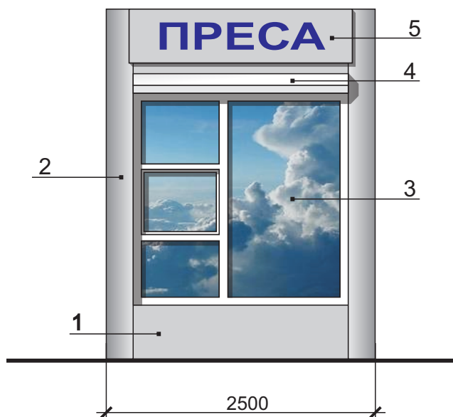
Боковий фасад. М 1:50
