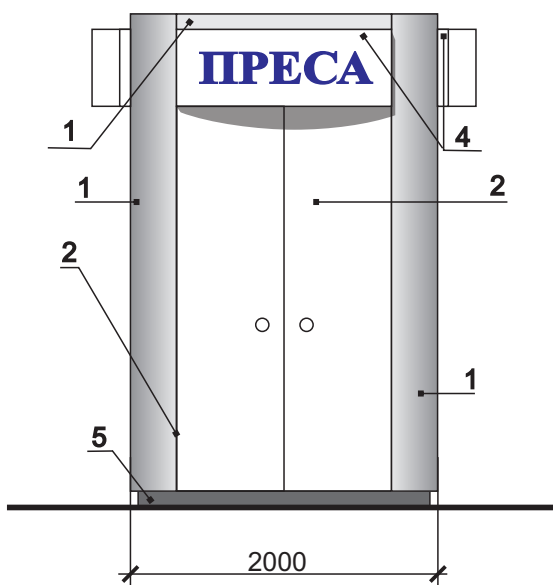
Тильний фасад. М 1:50
