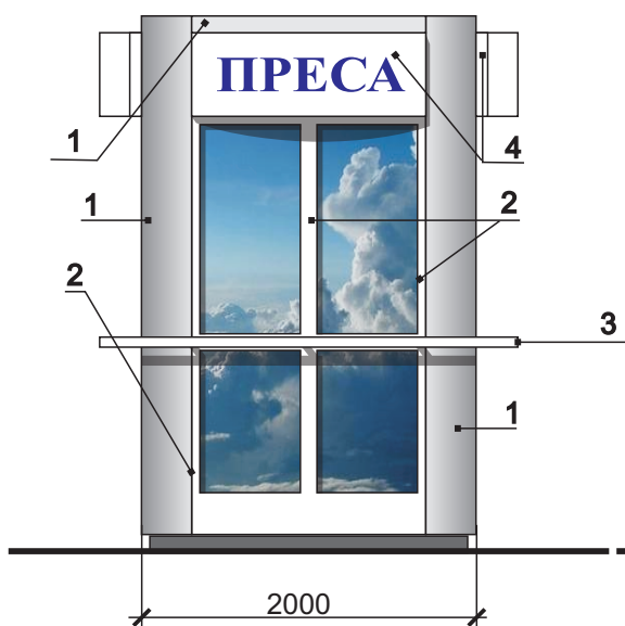
Боковий фасад. М 1:50
