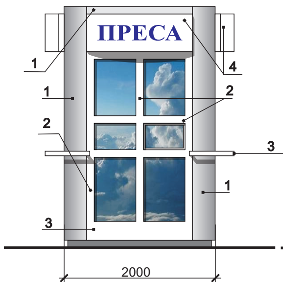
Головний фасад. М 1:50
