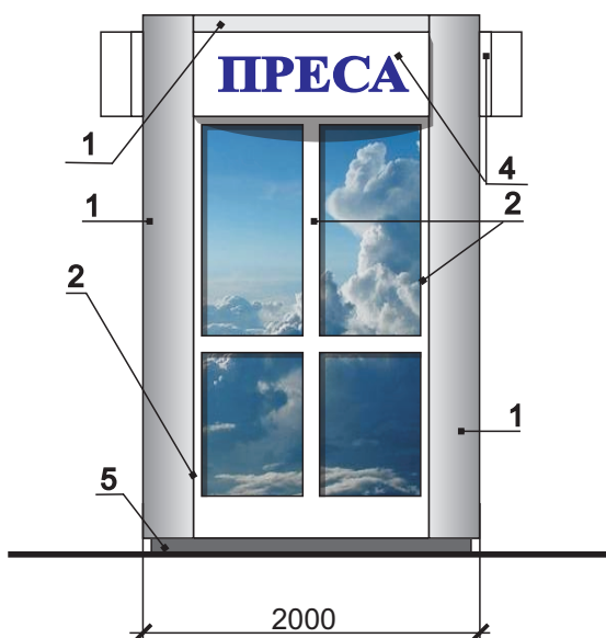
Боковий фасад. М 1:50
