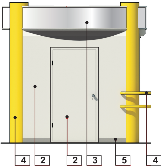
Фасад в осях А-Б. М 1:50.
