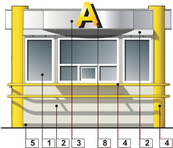
Фасад в осях 2-1. М 1:50.
