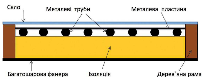
Розріз колектора
